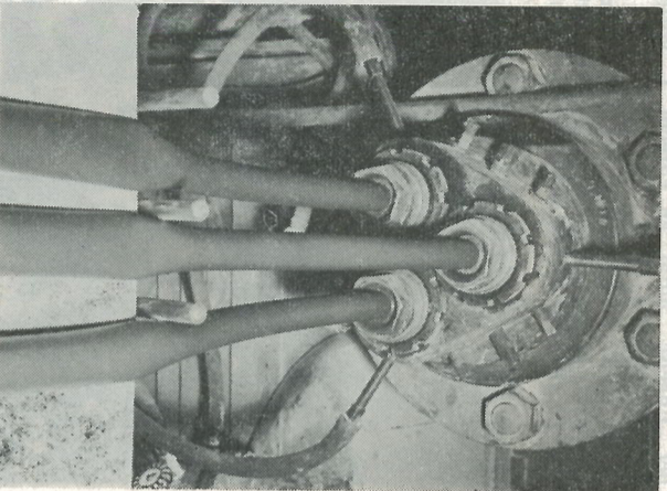
Spluitkop van de machine ter vervaardiging van het buismatieraal voor de Solex-potdichtbinnenband.
