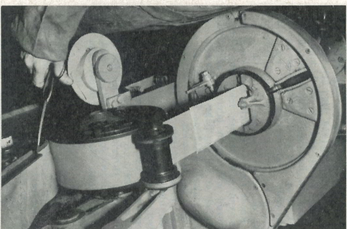
Machine om tussen de beide staal-draaithoepels van de Solex-buitenband het canvas aan te brengen (zelfde principe als bandlegmachine statorspelen in fabriek Utrecht).
