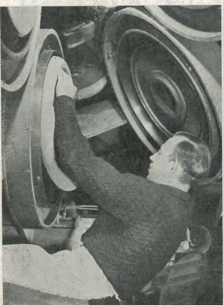
Geopende vulcaniseermatrijs voor buitenbanden
